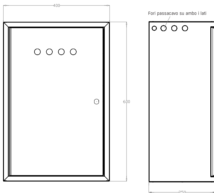
UNITÀ ALIMENTAZIONE E CONTROLLO SMRA-040
