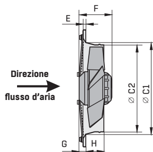
Dimensioni in mm versione AC
