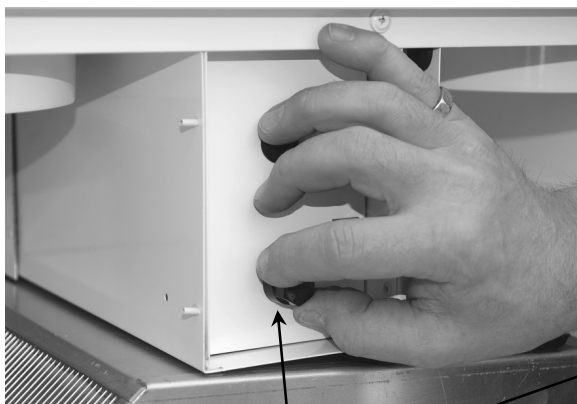
Ylikuumenemissuojan palautuspainike
