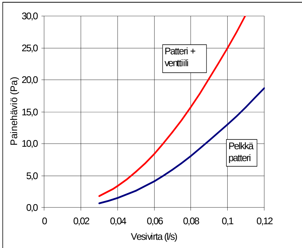
Kuva 4. Vesipatterin painehäviö
