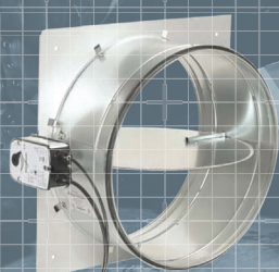
Cirkulært røgevakueringsspjæld (ETER) m. spring-return motor
